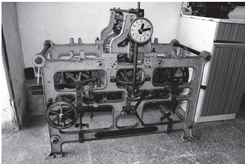
Torzo hodinového stroje v dílně zhotovitele v Oldřichově v květnu 2015, původní stav.
