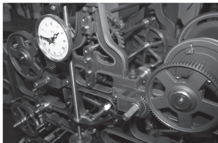
Převody natahování bití
