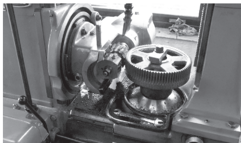
Výroba ozubených kol náťahu na odvalovací frézce v dílně zhotovitele.
