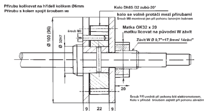
Technický výkres volnoběžného kola.
