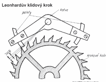
Náčrt krokového mechanismu Leonhardova kroku.
