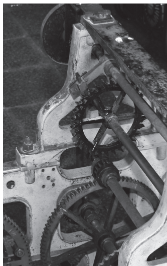
Krokové kolo s kotvou v původní přejaté podobě.
