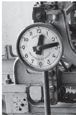
Rekonstrukce kontrolního ciferníku a jeho původní stav po zásahu OPP Vyškov.
