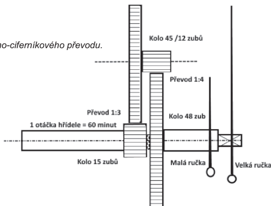
Ciferníkový převod 1:12 hodiny Potštát Franc X. Baitel. 1910
