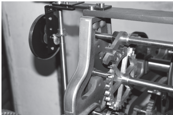
Krokové kolo po justáži s kotvou a kontrolním ciferníkem.
