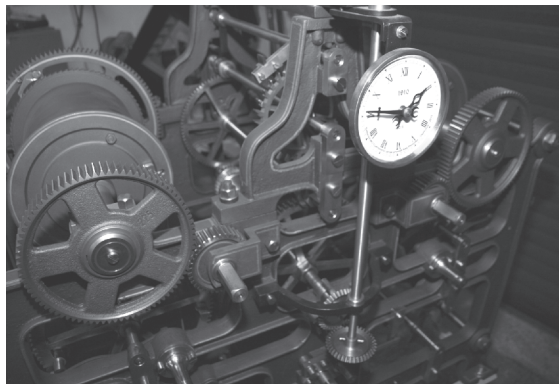
Pohled na kompletní hodinový stroj v dílně zhotovitele.
