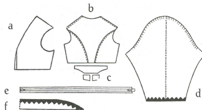
Krój szpencera z Orłowej, 1890 r. : a – przód, b – płat pleców, c – płatki fałdów, d – rekaw, e – pasek, f – połowa kołnierza.
